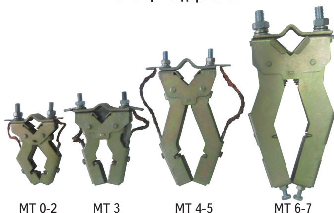
Рис. 2. Щеткодержатель
